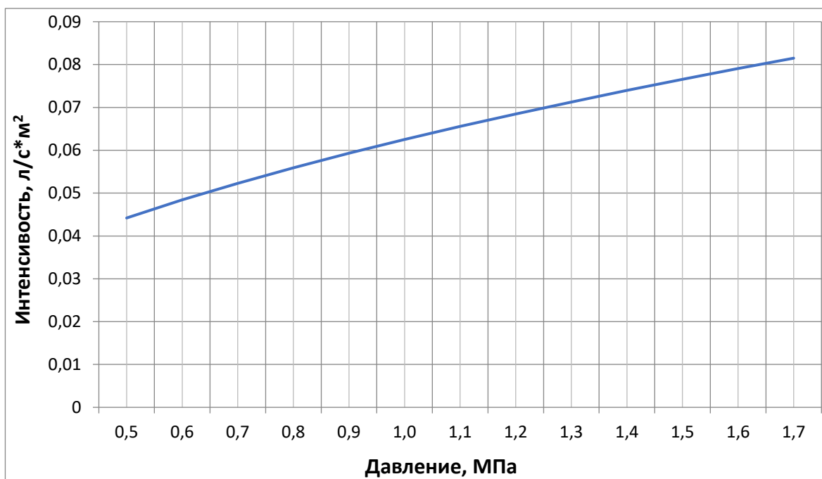
График зависимости интенсивности орошения от давления на площади 16 м 2 , защищаемой одним оросителем с высоты 2,5 м
